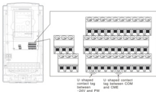
Рис. 3-7 U-образный контакт
