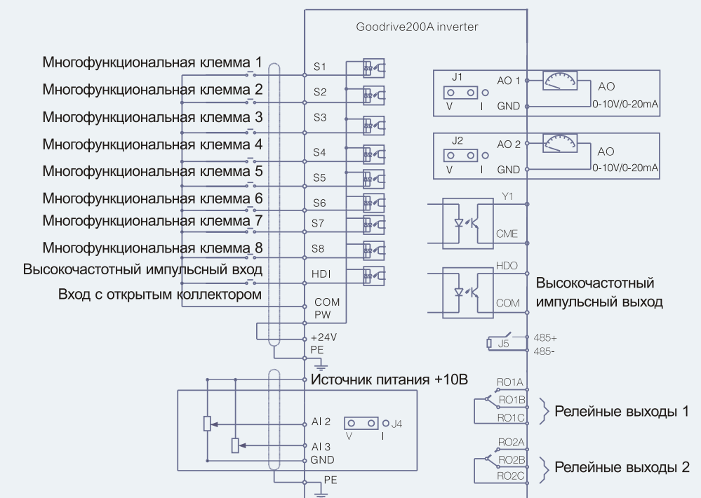
Схема подключения цепи управления
